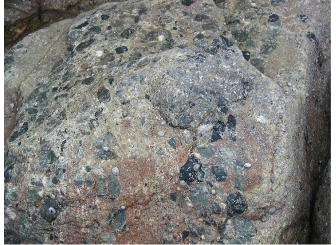
Fig.80 : C : Conglomérat de base de la Série des Sévignés (2004)
