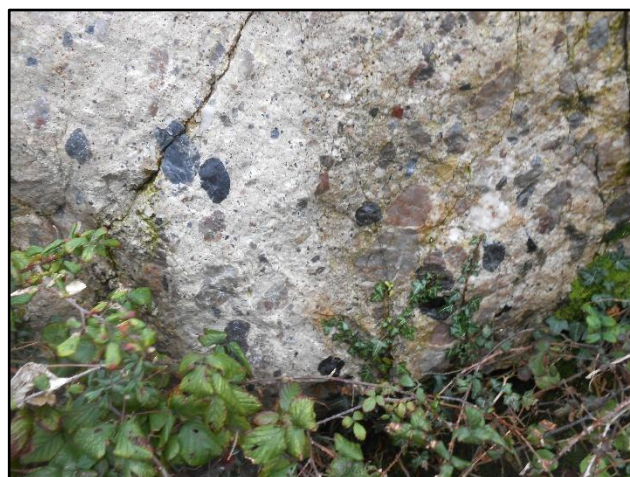
Fig.50 : Poudingue clair, à galets multicolores, en falaise
