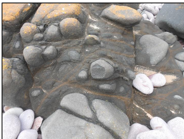
Fig.47 : Altération en boules de la dolérite
