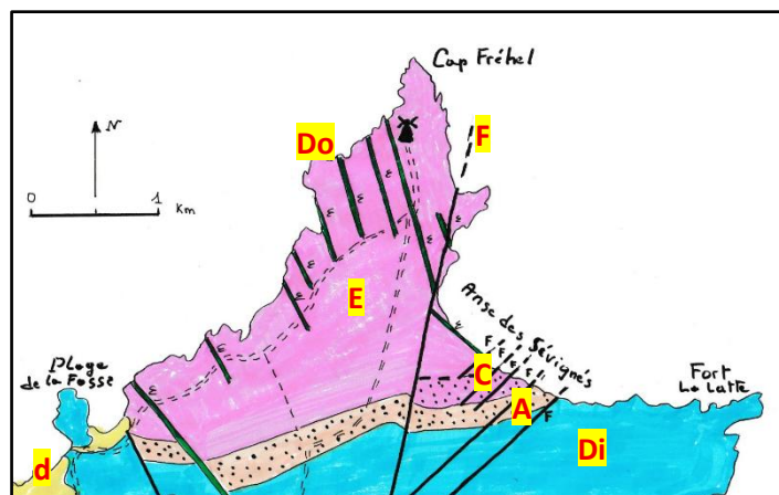
Fig.71 : Carte géologique du Cap-Fréhel (carte BRGM modifiée)
