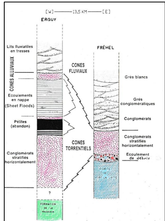
Fig.6 : Corrélation stratigraphique des faciès des séries d'Erquy-et du Cap Fréhel (d'après O Dauteuil, 1985)
