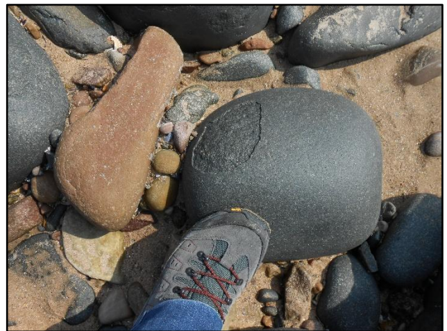
Fig.68 : Altération en « pelure d'oignon » (photo GM2019)
