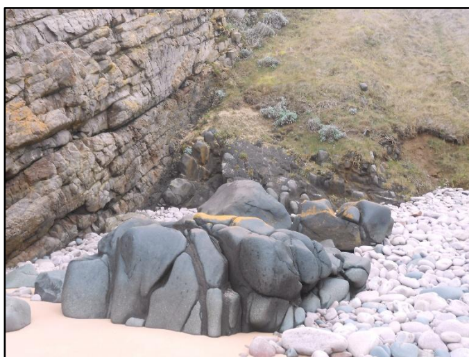
Fig.46 : Filon de dolérite recoupant le grès
