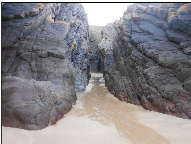
Fig.45 : Couloir étroit se terminant par une grotte
