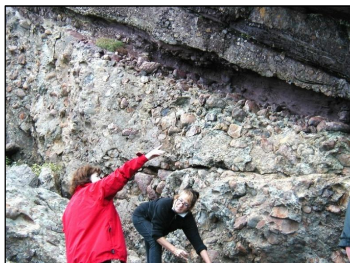
Fig.75 : A : Conglomérat de base (2004)
