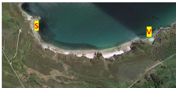
Fig.70 : Anse des Sévignés (photo satellite Google Earth 2020)
