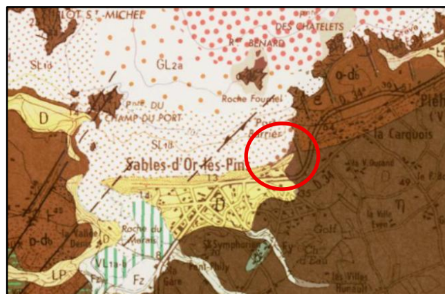
Fig.49 : Site de Port-Barrier (carte géologique 1/50000 °BRGM)
